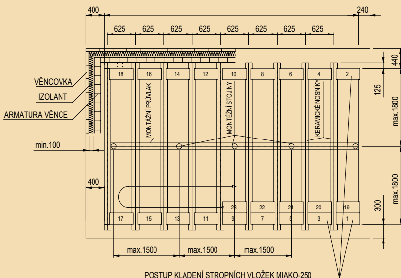
POSTUP KLADENÍ STROPNÍCH VLOŽEK MIAKO-250
