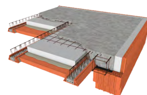
Stropní systém Hurdís
