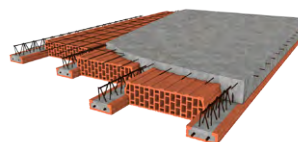
Stropní systém Miako
