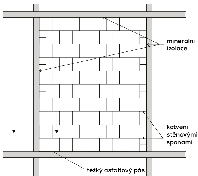
Pružné připojení ke skeletové konstrukci
