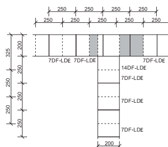
T převazba 200/200 mm 7DF/7DF
