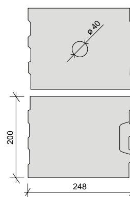
Převazba rohu 200/200 mm 7DF/7DF
