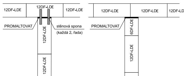
1. vrstva
