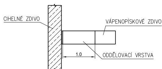
ŘEZ A-A
