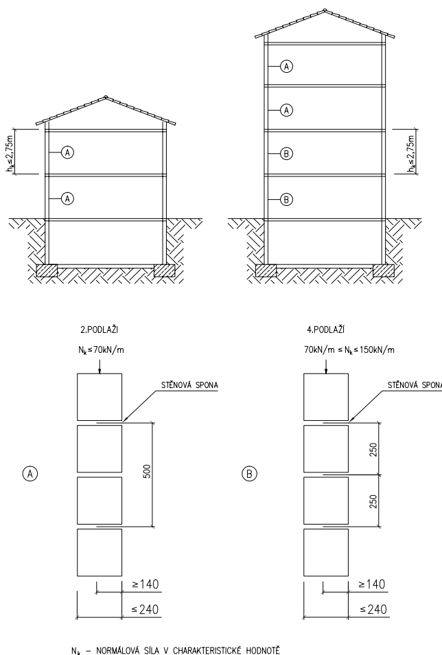
Tupé spoje
