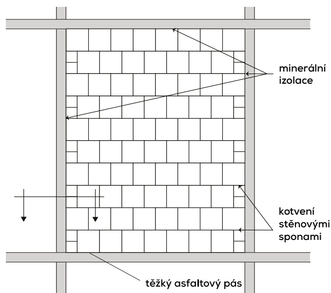
Pružné připojení ke skeletové konstrukci
