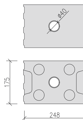
Vazba zdiva z 6DF-LDZHE
