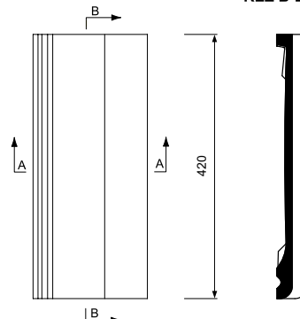
ŘEZ B-B
