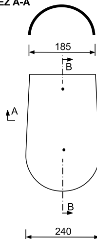
ŘEZ A-A
